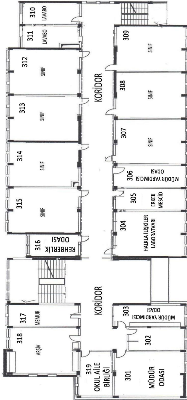
1. KAT PLANI
